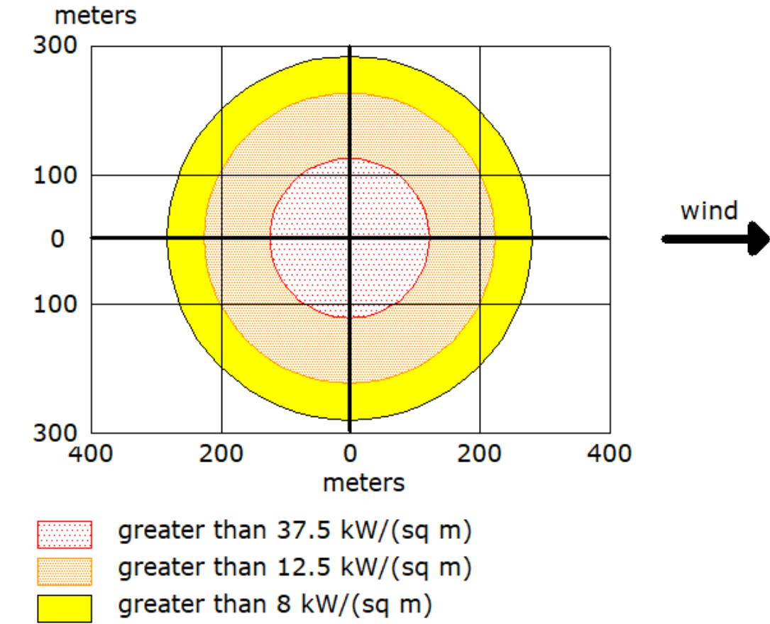
Imagen QTC - B - 05. Bola de fuego por explosion tipo bleve - escenario 02
