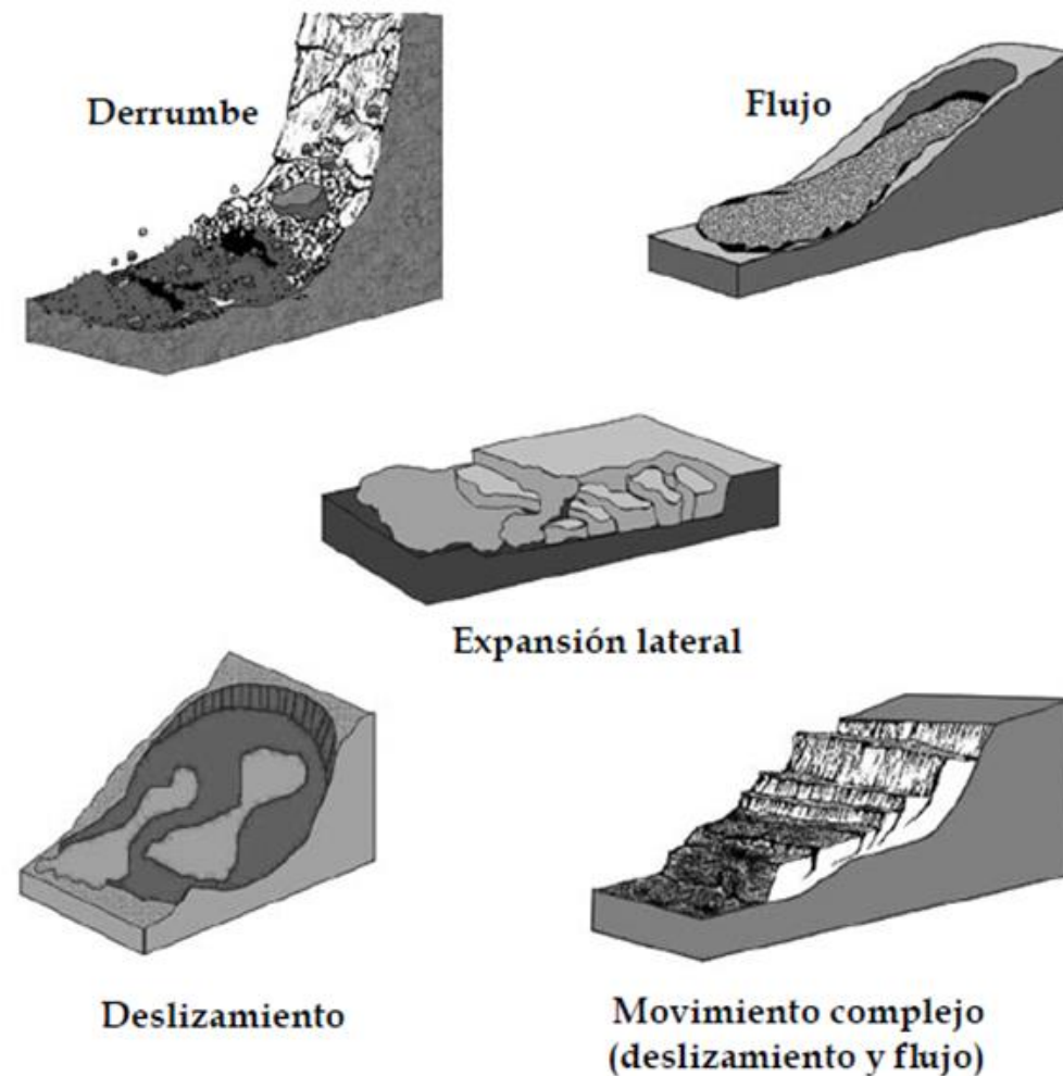
Imagen GEO-A-1. Tipos de procesos de remoción en masa.
