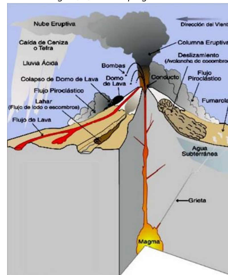
Imagen GEO-D-1. Los peligros volcánicos
