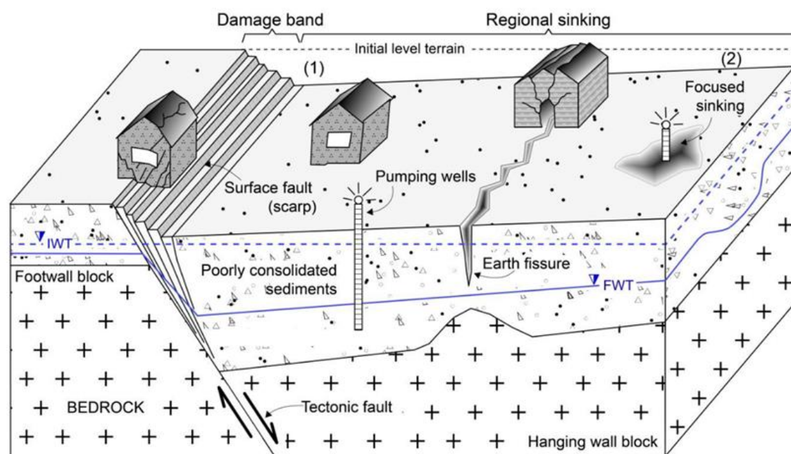
Imagen GEO-C-1. Subsistencia diferencial estructuralmente-controlada
