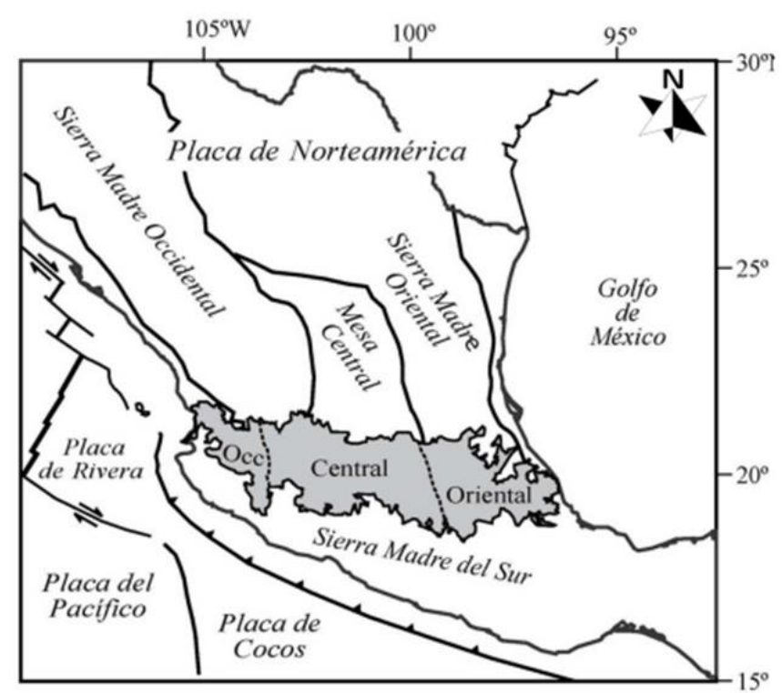
Imagen GEO-B-4. Descripción tectónica del centro
