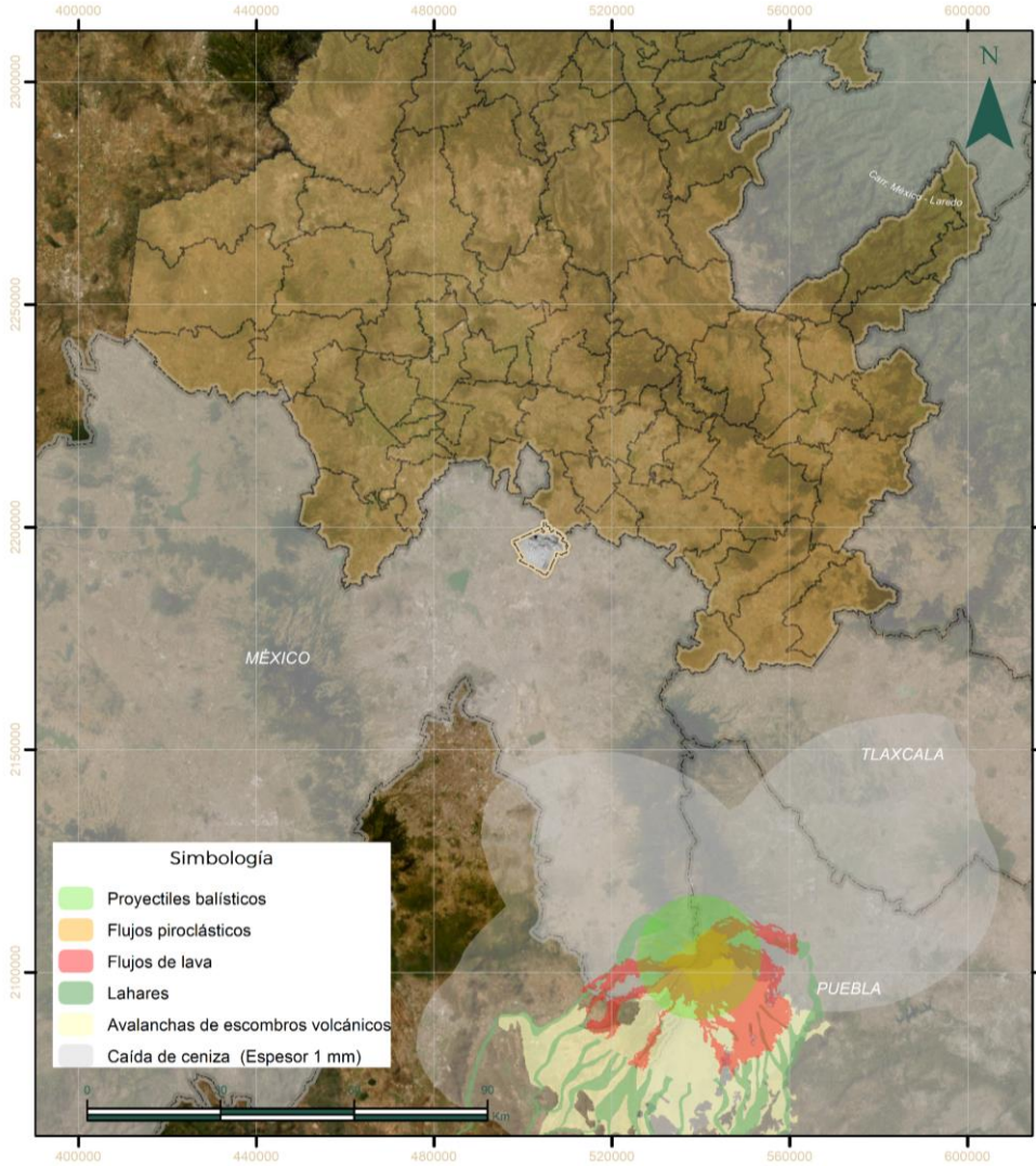
Imagen GEO-D-4. Mapa de peligros volcánicos del Popocatepetl y su influencia en Tizayuca
