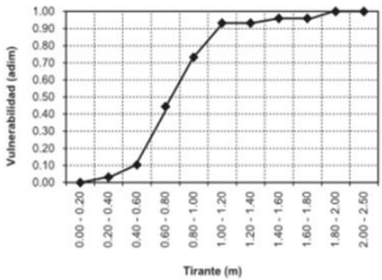
Función de vulnerabilidad para vivienda tipo III
