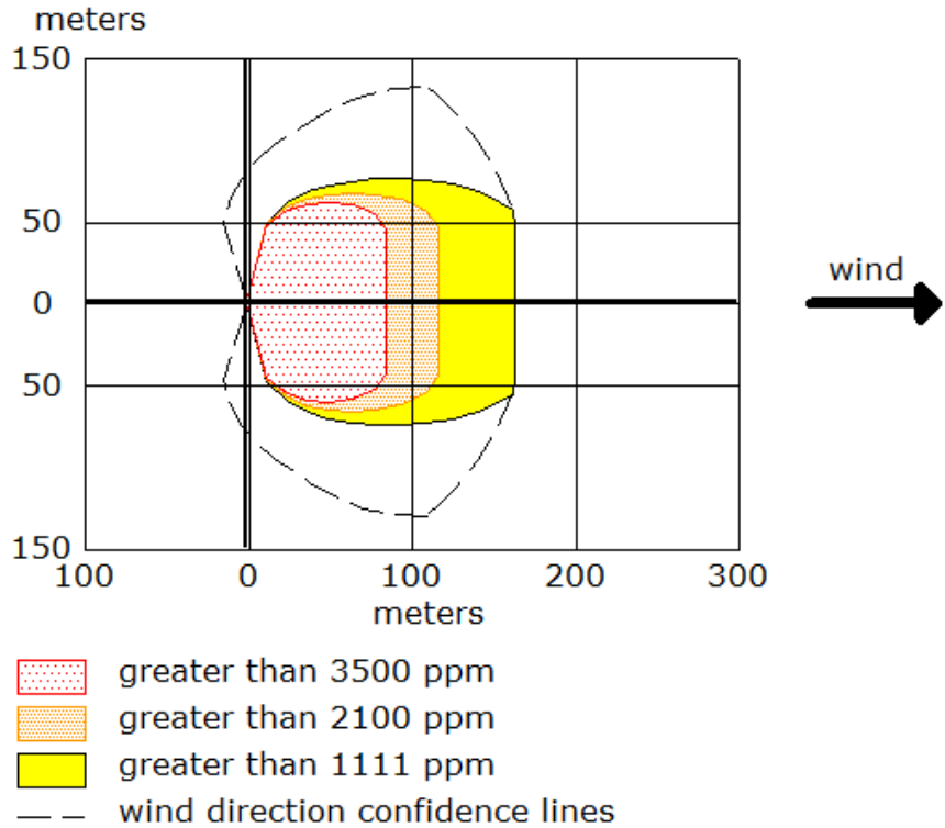
Imagen QTC - B - 05. Nube inflamable de tipo flash fire - escenario 01
