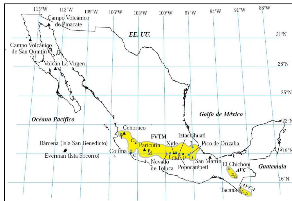
Imagen GEO-D-2. Ubicación de los principales volcanes dentro de la FVTM
