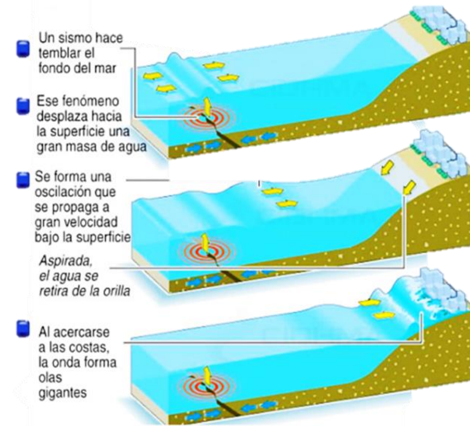
Imagen GEO-C. Formación de un Tsunami.
