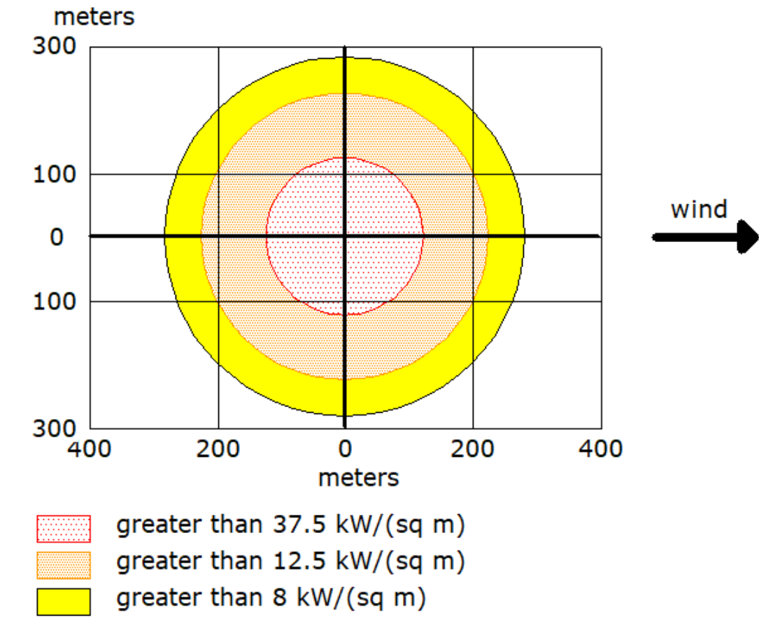
Imagen QTC - B - 05. Bola de fuego por explosion tipo bleve - escenario 03
