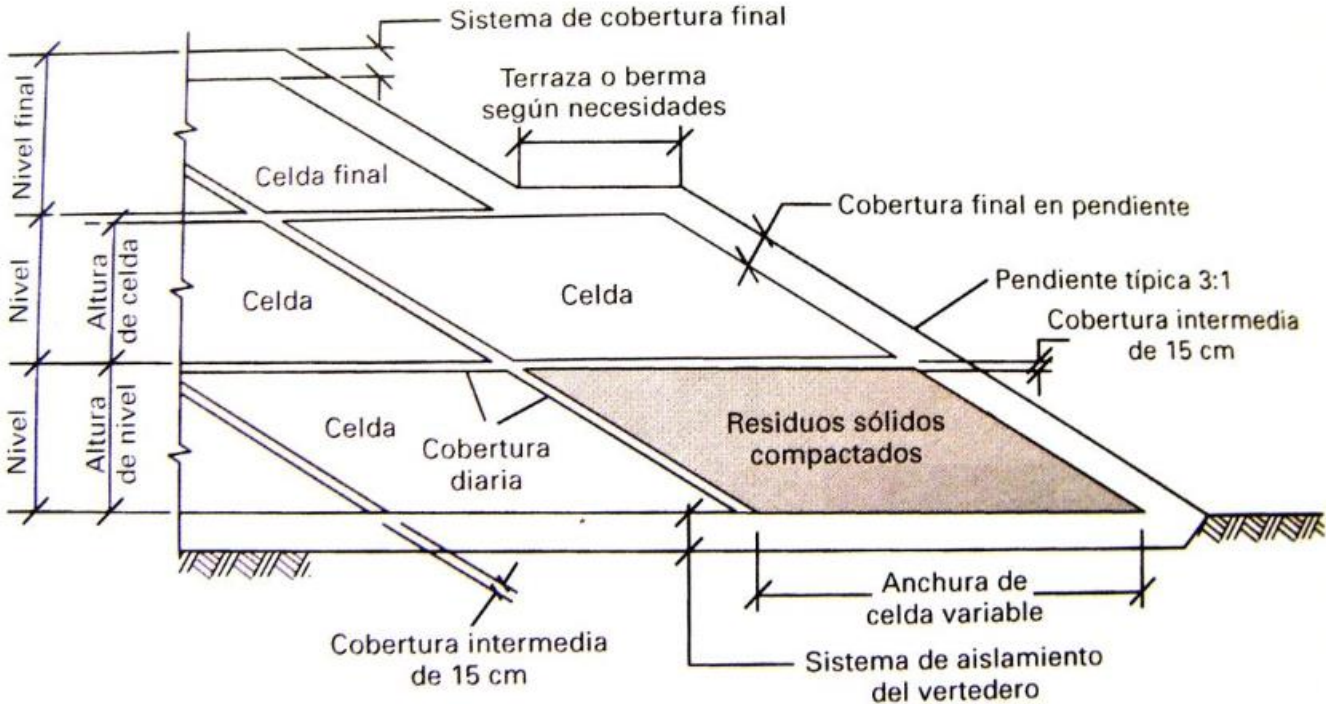
Imagen ECO-A-5. Secciones de un relleno sanitario controlado
