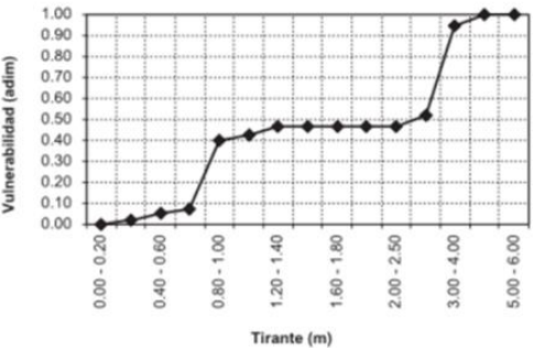
Función de vulnerabilidad para vivienda tipo IV
